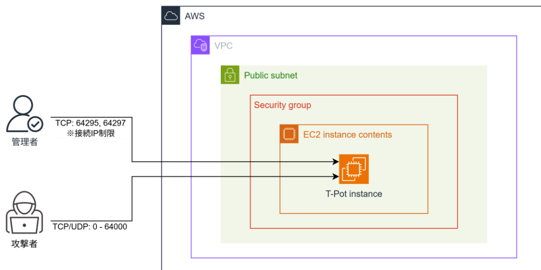
図 3：AWS 上のハニーポット配置構成図
